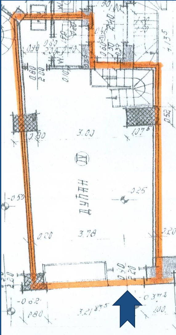
Основа приземља
